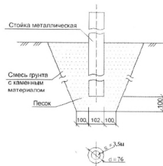
Пример установки стойки в грунт
