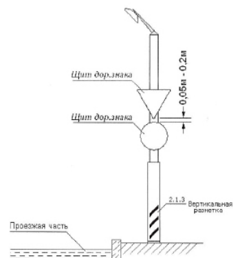
Установка на конструктивно выделенных направляющих островках или островках безопасности
