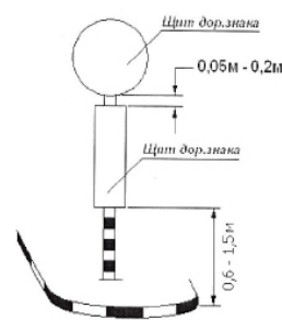
Пример установки стойки в грунт
