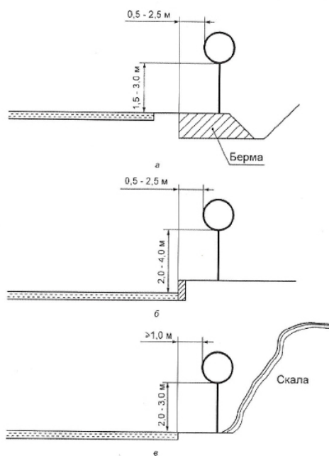
а - вне населенных пунктов; б - в населенных пунктах; в - на обочине в стесненных условиях
